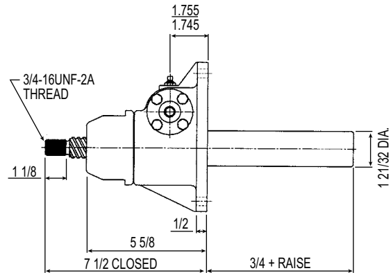
Upright: M-78021
