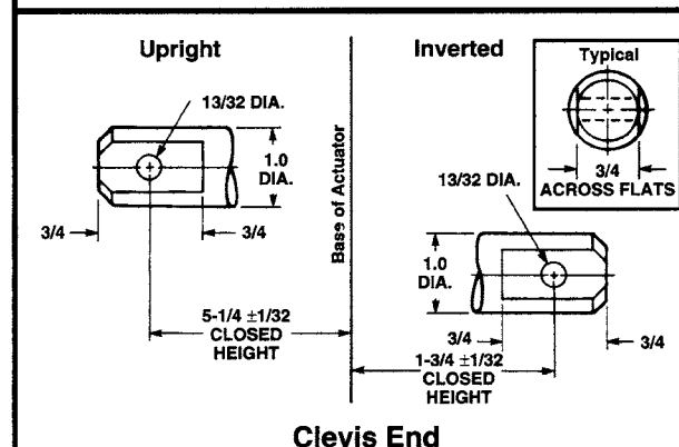
Clevis End
