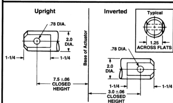
Clevis End
