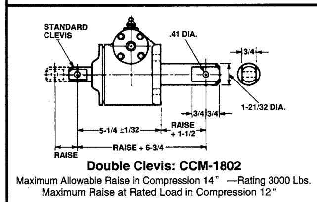
Clevis End
