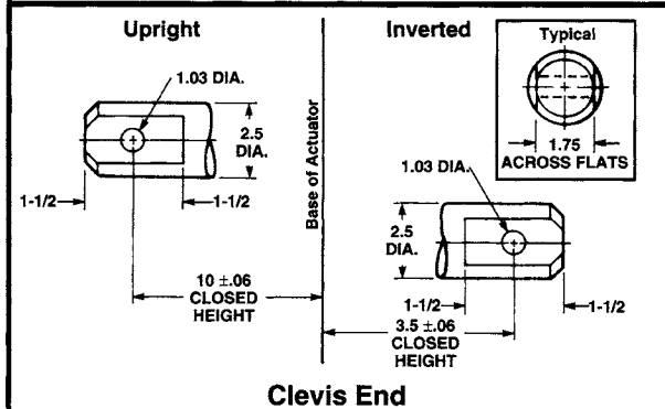
Clevis End
