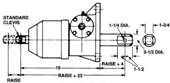
Clevis End (Optional) SK2800-4-20A
