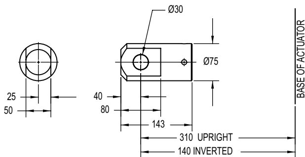
Clevis End G9020-11
