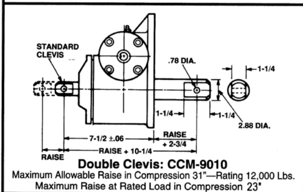
Clevis End
