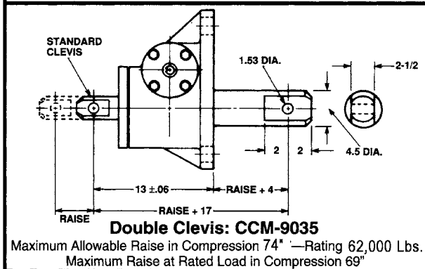
Clevis End
